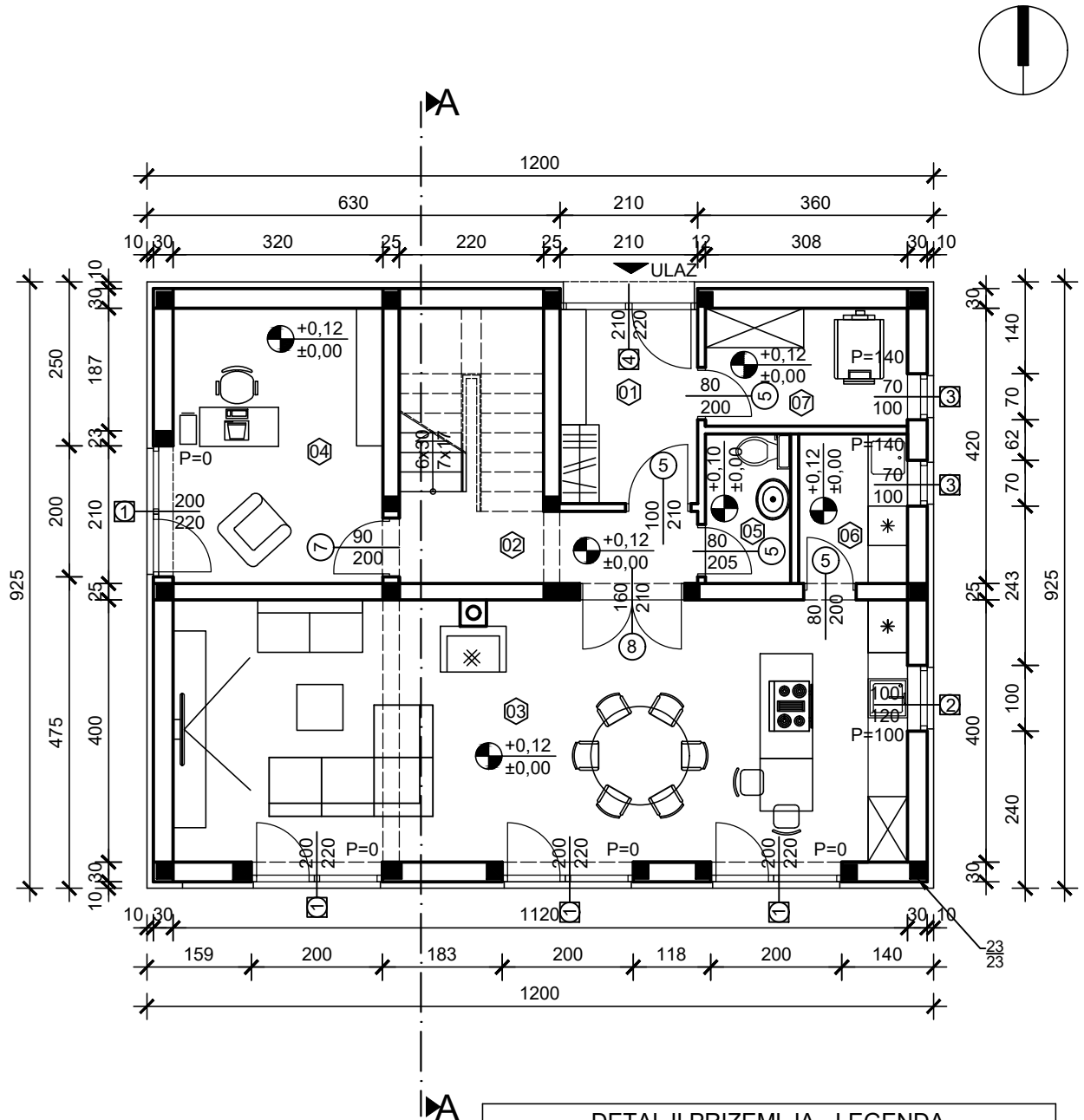
DETALJI PRIZEMLJA - LEGENDA
