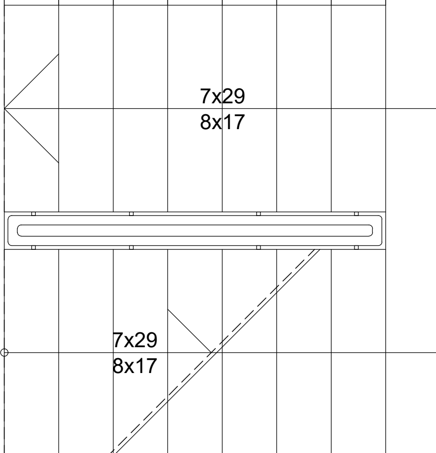
TLOCRT DVOKRAKOG STUBIŠTA MJ. 1:20
